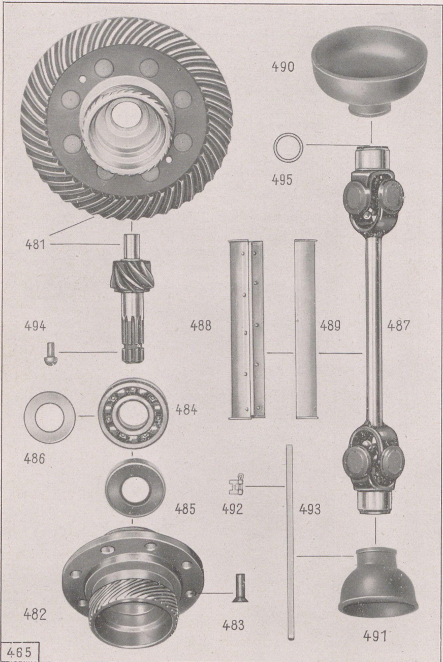
Tafel 17, Gruppe H: c) Hinterachstriebwerk
