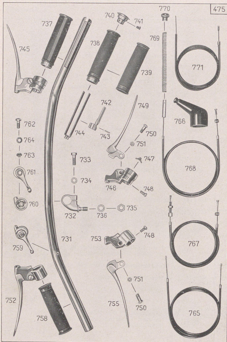
Tafel 27, Gruppe R: gj Lenker und Handbetätigungen mit Seilzügen
