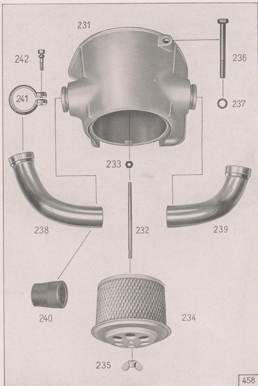
Tafel 10, Gruppe M: f) Vergaser, Luffilter und Saugleitungen
