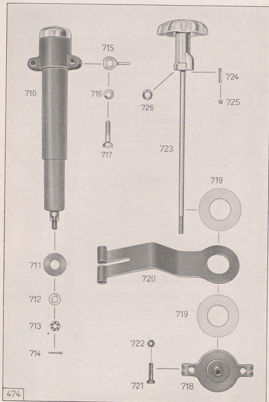
Tafel 26, Gruppe R: f) Vordergabel, Stoßdämpfer, Steuerungsdämpfer
