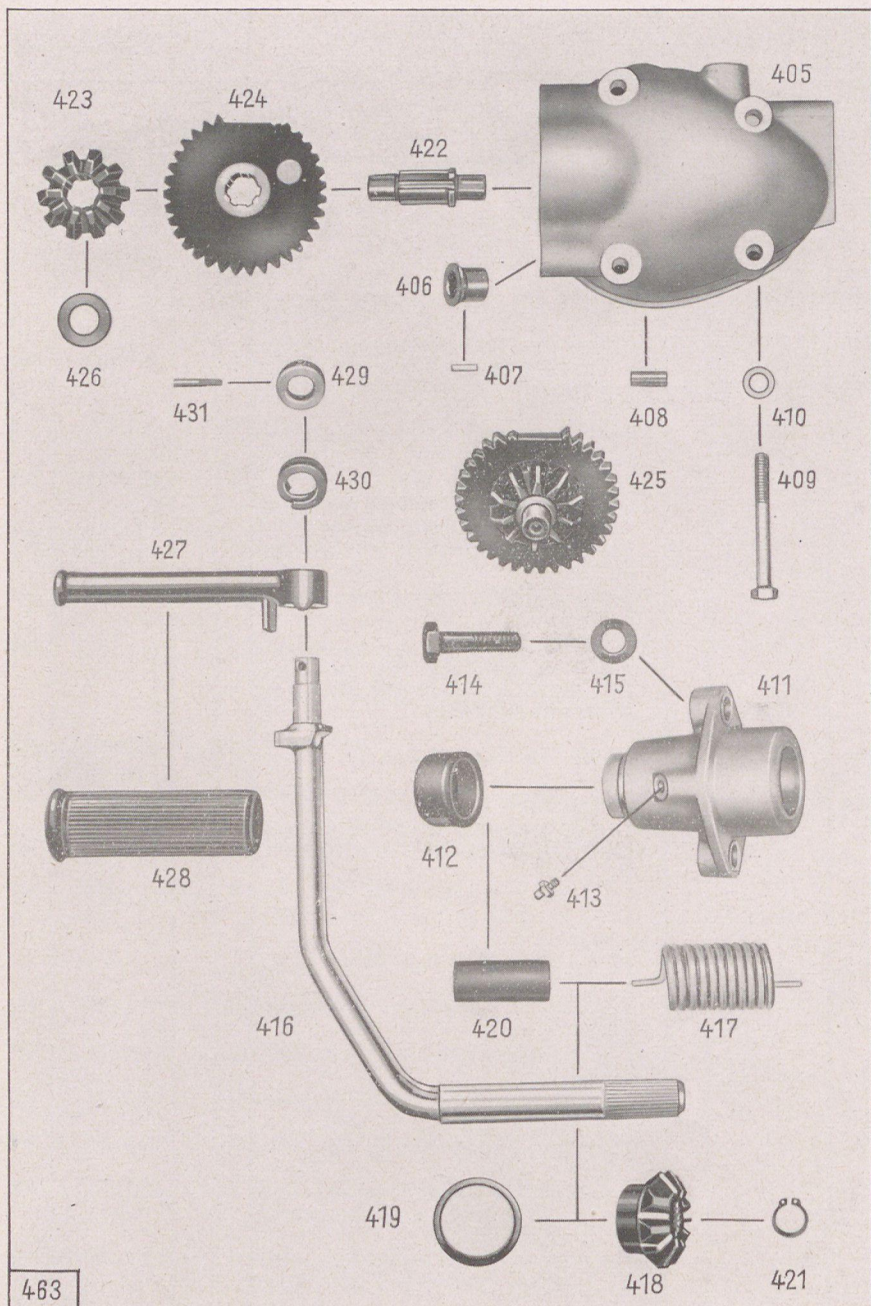
Tafel 15, Gruppe G: e) Anwerfer
