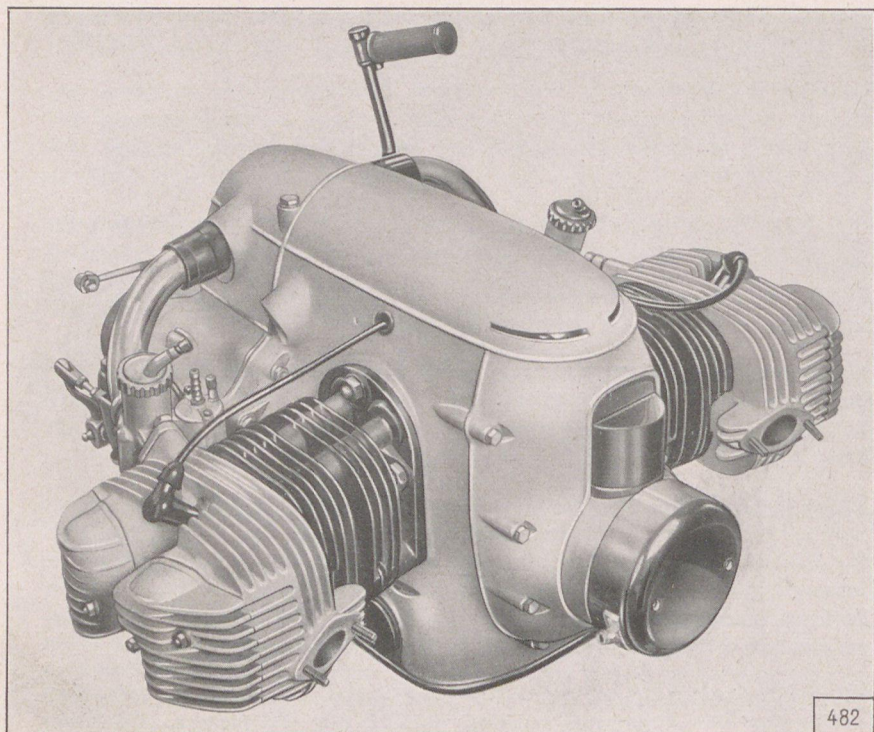
Tafel 1, Gruppe M: a) Motor (Zusammenbau)
